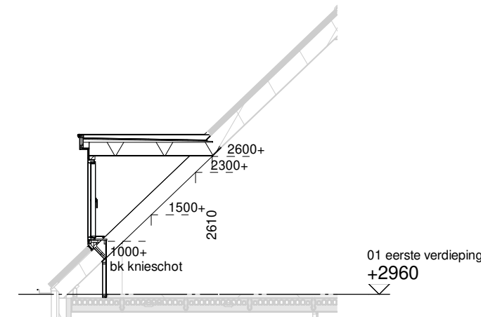
Doorsnede schaal 1:100
